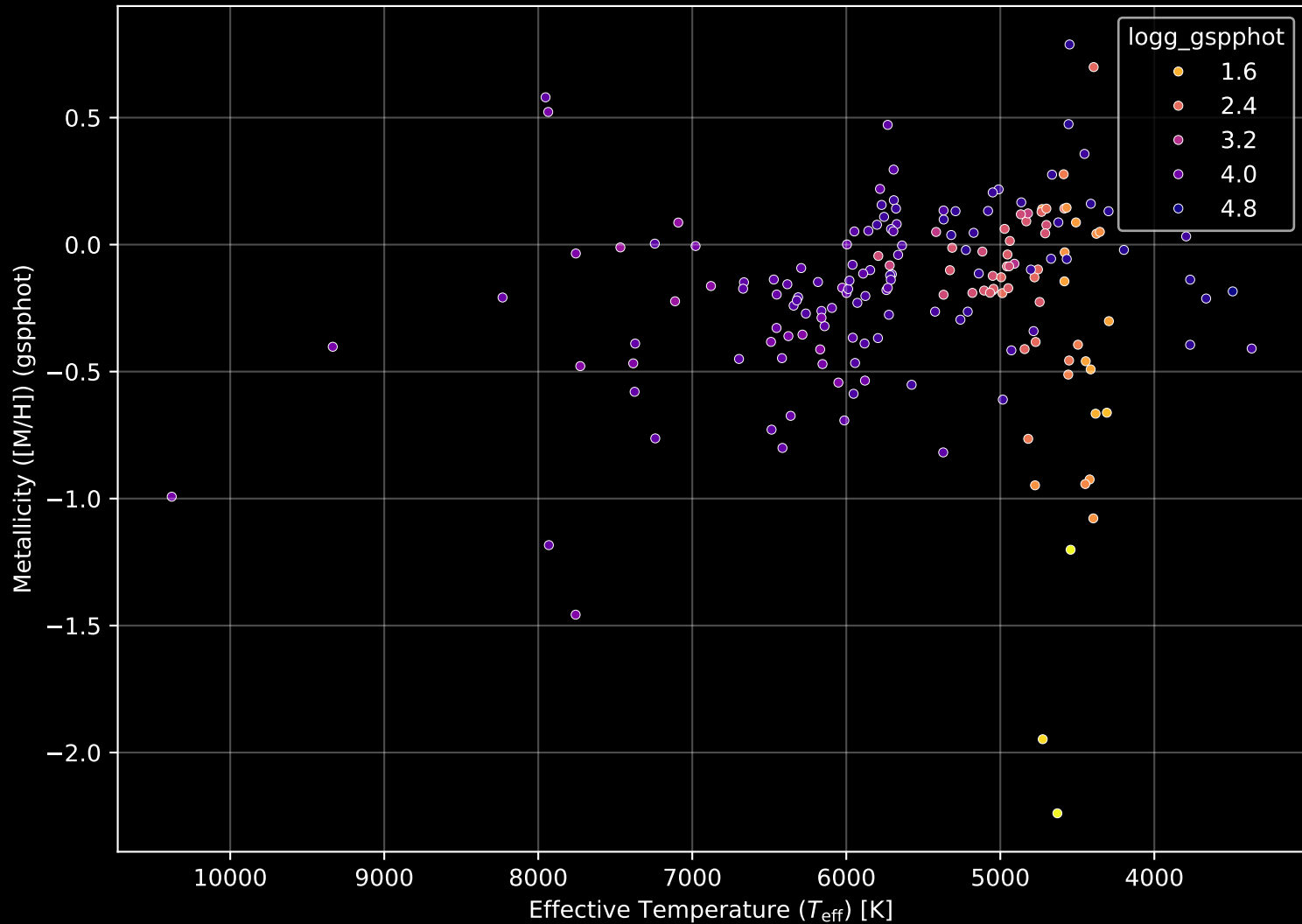
APOGEE DR17 Field: [CVZTILE_101+20_btx] Stellar Population Parameters (n= 181)
